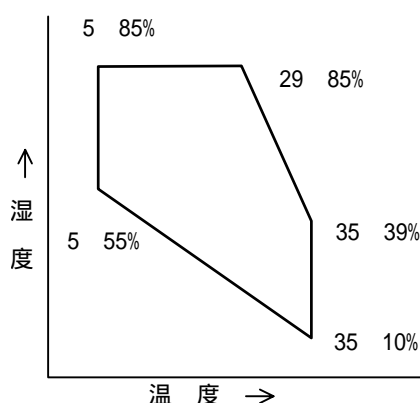
図4 温度-湿度図
