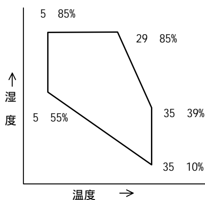
温度-湿度图
