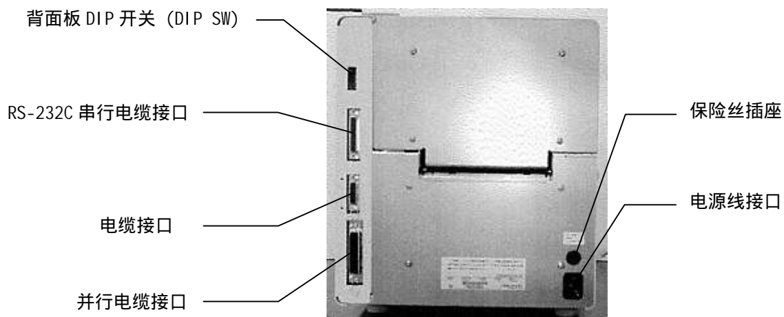
图 6 背面图
